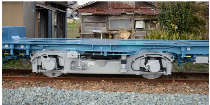
コキ73台車 FT16
